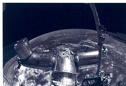
国際宇宙ステーション「きぼう」日本実験棟と地球 ©JAXA/NASA
